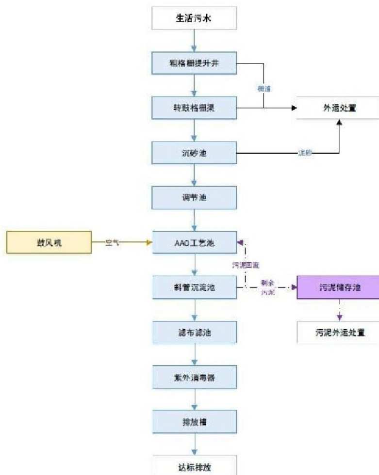
图 5-2 污水处理厂处理工艺流程图
