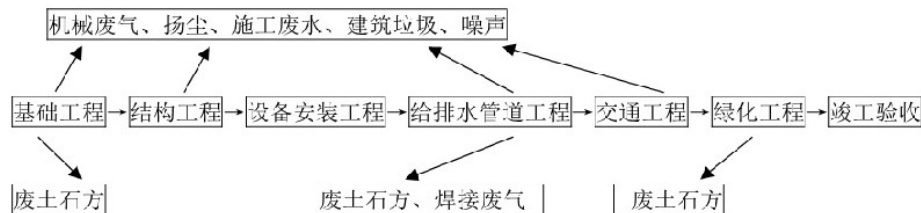
图 5-1 施工期产污工艺流程图
