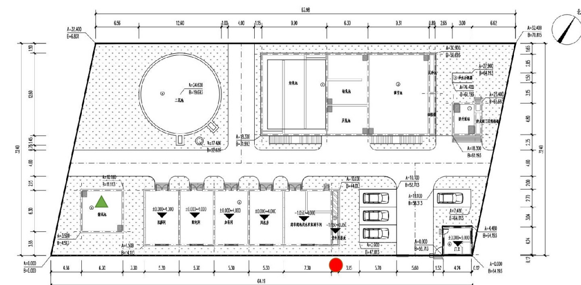
附图 4 项目平面布置图
