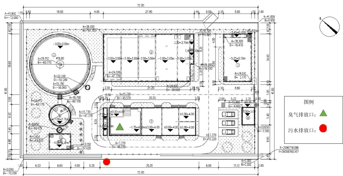
附图 4 项目平面布置
