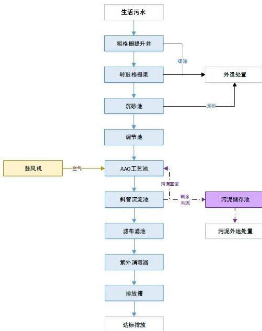
图 5-2 污水处理厂处理工艺流程图
