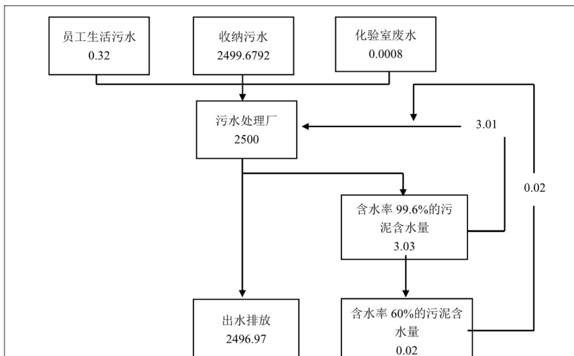
图 5-3 项目运营期日用水水平衡图 单位：t/d
