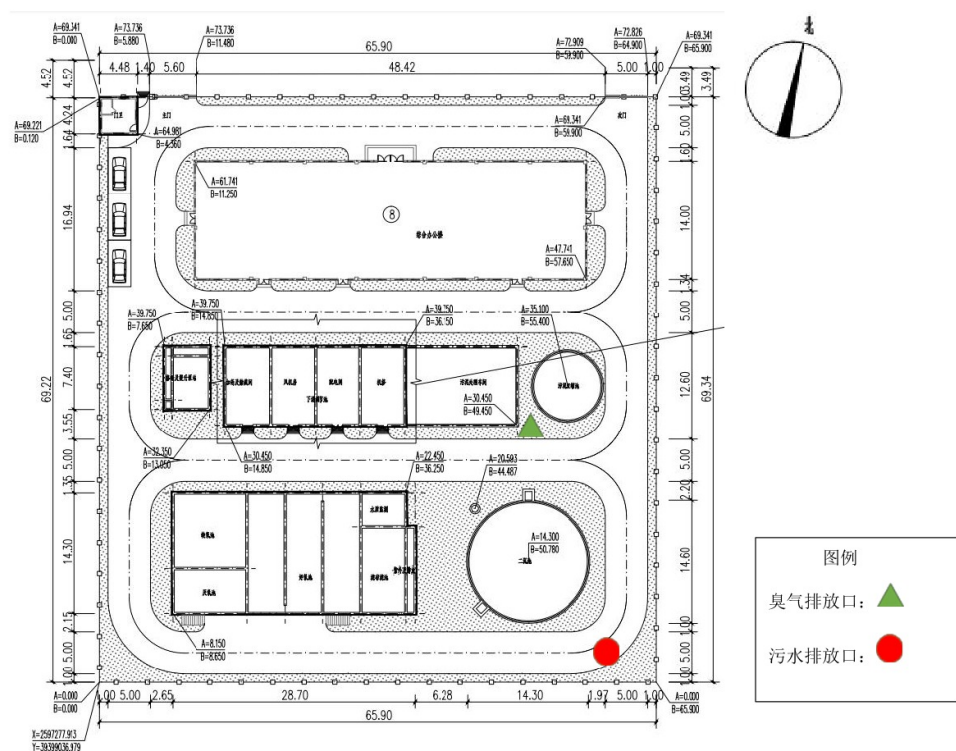
附图 4 项目平面布置图
