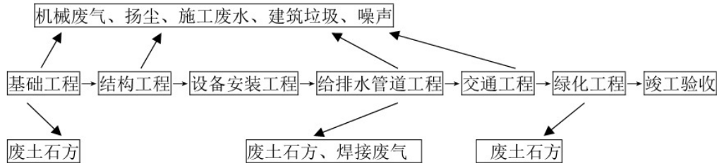
图 5-1 施工期产污工艺流程图
